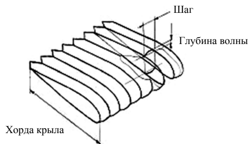
Рис. 5. Модель крыла с волнистой поверхностью
