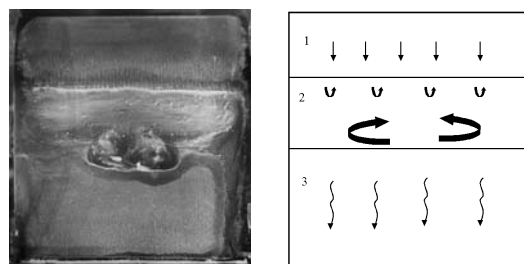
Рис. 6. Визуализация течения и ее трактовка над крылом с гладкой поверхностью (угол атаки \alpha = 0^\circ , скорость набегающего потока V_\infty = 12 м/с; Re = 1,7 \cdot 10^5 ): 1 – область ламинарного течения; 2 – область отрывного пузыря; 3 – область турбулентного течения [21]
