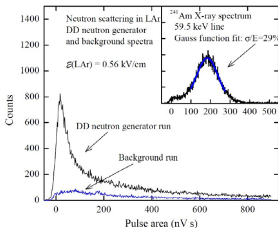
Рис. 2. Амплитудное распределение сигнала двухфазного КЛД в измерительных заходах, когда нейтронный генератор был включен (DD neutron generator run) и выключен (Background run). Во вставке показано амплитудное распределение сигнала, вызванного рентгеновским излучением от источника ^{241}\text{Am} в калибровочном заходе
