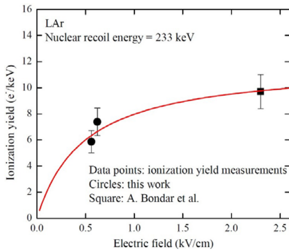
Рис. 5. Ионизационный выход ядер отдачи в жидком Ar при 233 кэВ, измеренный в данной работе и в работе [7], как функция электрического поля. Также показана аппроксимация данных теоретическими моделями Яффи (при \eta = 0 и \eta = 6,3 эВ) и выражением (2). Все три кривые совпадают
