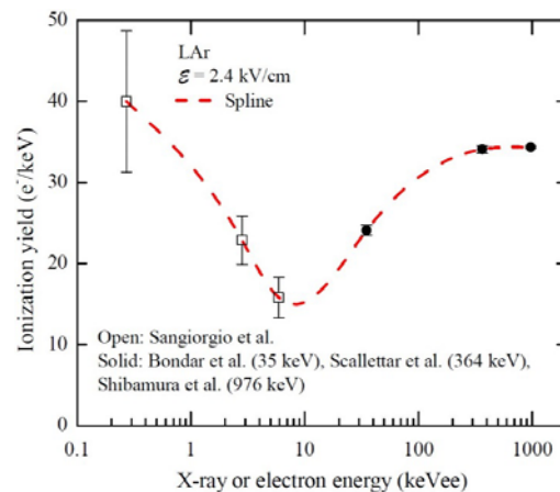
Рис. 7. Ионизационные выходы электронов отдачи в жидком Ar при электрическом поле 2,4 кВ/см как функция энергии. Данные взяты из Sangiorgio et al. [29] (при 0,27, 2,8 и 5,9 кэВ), из Bondar et al. [14] (при 35 кэВ), из Scallettar et al. [30] (при 364 кэВ) и из Shibamura et al. [31] (при 976 кэВ) и аппроксимированы сплайн-кривой (рисунок приводится по: [14])
